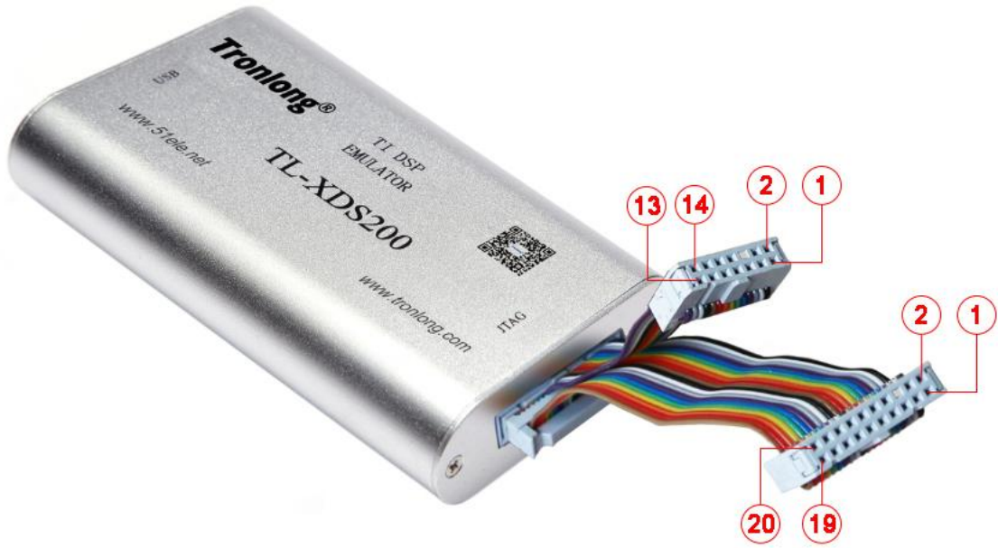
图 4 20-20-14pin JTAG 转接排线
